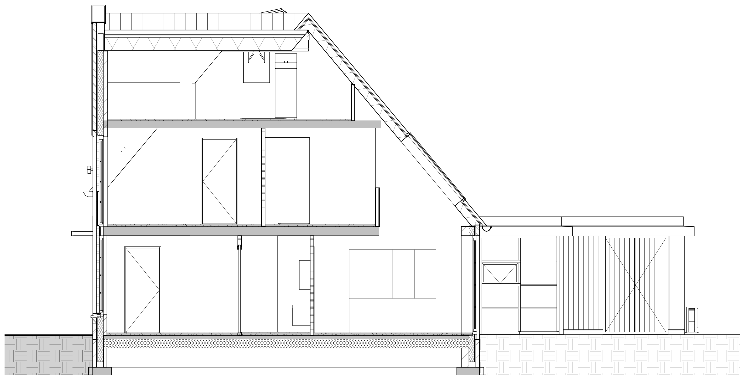
Doorsnede VK-8
